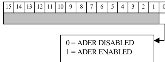
Fig. 3.16: ENABLE ADER Register
